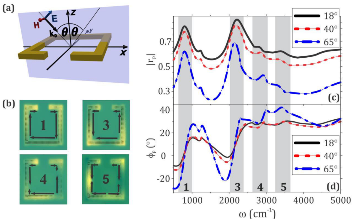
Slika 4.5: (a) Šema upadne xz -ravni i p-polarizovanog upadnog polja. (b) Raspodele struja u prstenovima i komponente |E_z| polja na rezonantnim učestanostima pri upadnom uglu od 65^\circ . (c) Apsolutna vrednost i (d) faza koeficijenta refleksije u datoj konfiguraciji.
