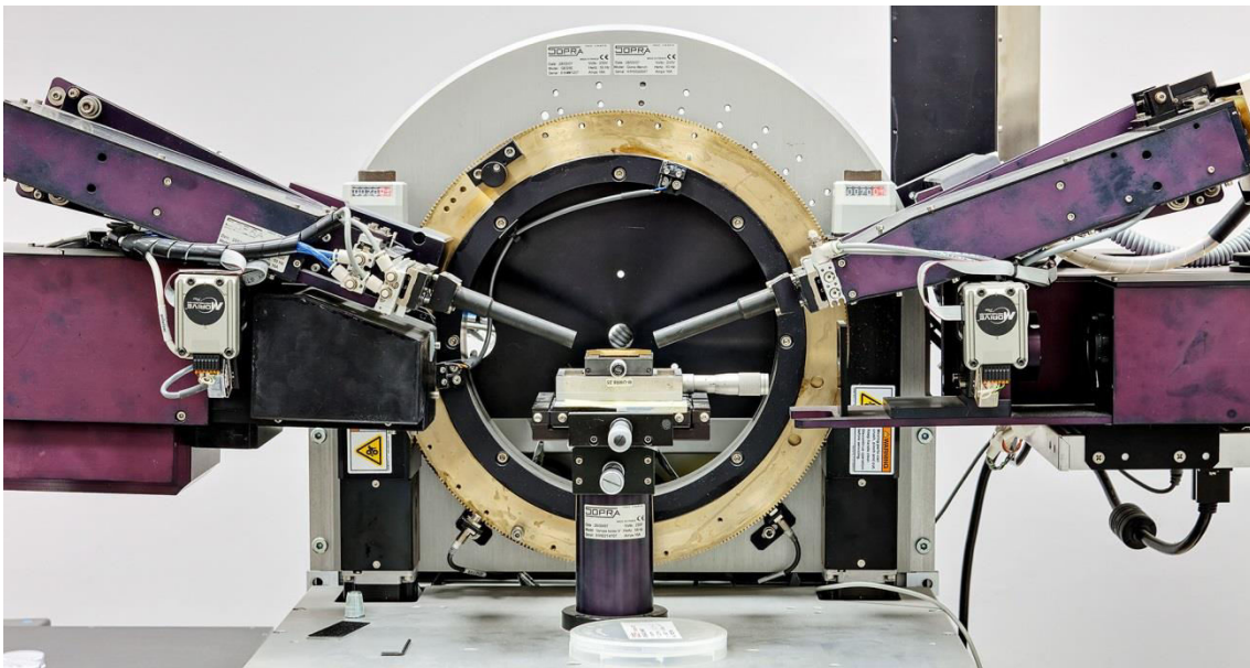
Slika 2.10: SOPRA GS5 IR spektroskopski elipsometar u laboratoriji Centra za čvrsta stanja i nove materijale, Instituta za fiziku u Beogradu.
