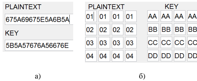
Слика 4.5. Визуелна репрезентација конфигурирања улазних параметара за DES и AES алгоритме у COALA систему
