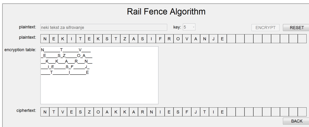
Слика 5.7. Екран за визуелну репрезентацију Rail Fence алгоритма у COALA систему моноалфabetски алгоритам и притисне дугме START .
